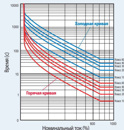
<Характеристика обратно-зависимой выдержки времени>
