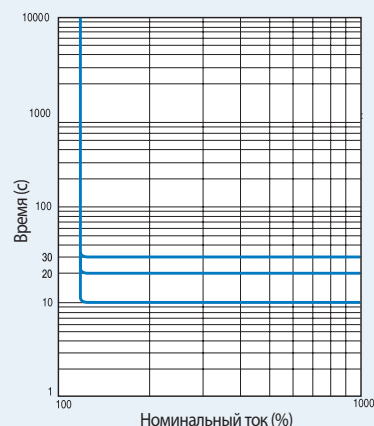
<Характеристика независимой выдержки времени>
